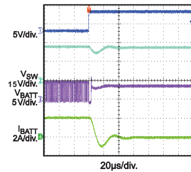
En Off V_{BATT} = 7.2V
