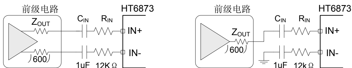
图 1 (1) 差分输入;
